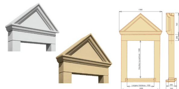
LUCARNE À FRONTON 40° 1350 X 900 MM
