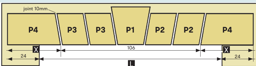
Linteau 120-140
