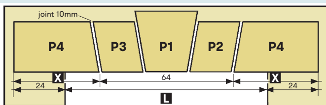
Linteau 80-100
