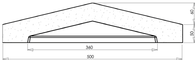
CHAPEAU DE PILIER CHEVERNY POINTE DE DIAMANTS , Adapté pour pilier sans chapiteau 500 X 500 X 110 MM
