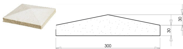
CHAPEAU DE PILIER CHEVERNY POINTE DE DIAMANTS 300 X 300 X 60 MM
