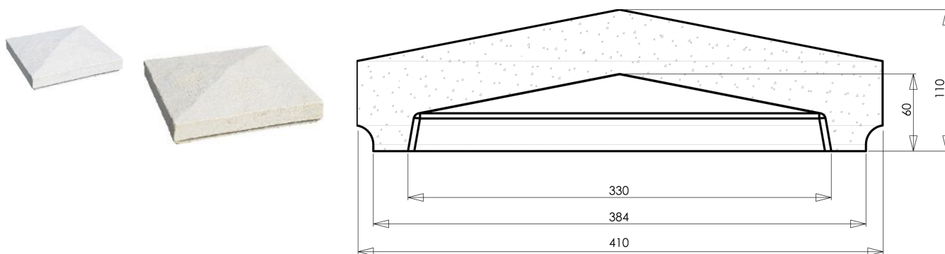
CHAPEAU DE PILIER CHAUMONT POINTE DE DIAMANT 410 X 410 X 110 MM :
