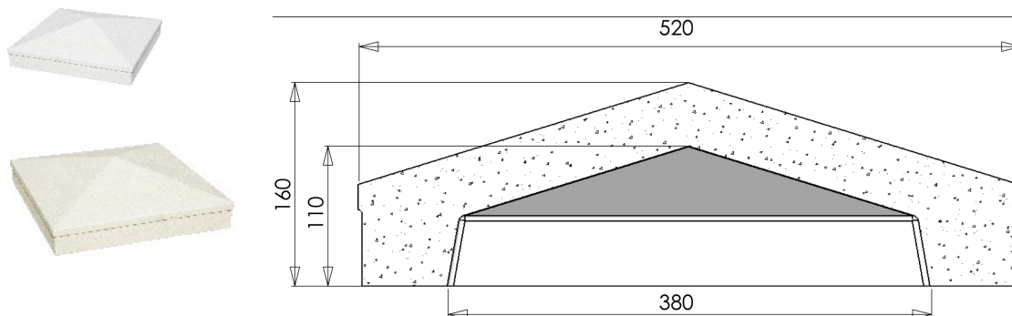
CHAPEAU DE PILIER AMBOISE POINTE DE DIAMANT 520 X 520 MM :
