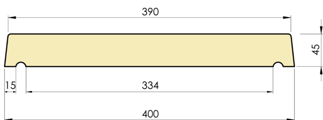
CHAPEAU DE PILIER PIERRE LISSE PLAT 400 x 400 MM
