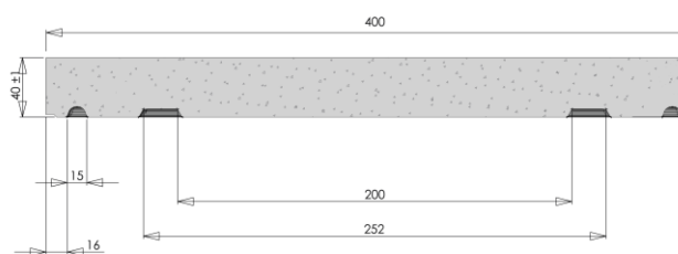
CHAPEAU DE PILIER PLAT 400 x 400 MM
