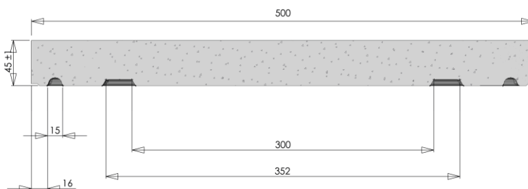
CHAPEAU DE PILIER PLAT 500 x 500 MM
