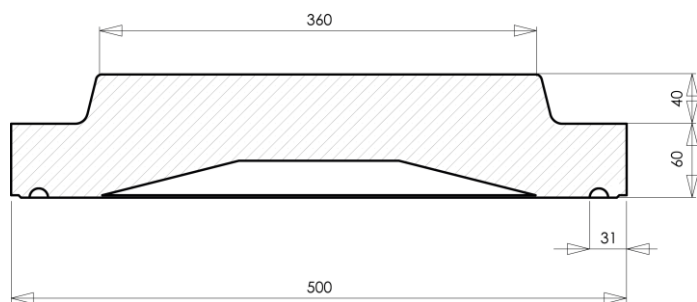
CHAPEAU DE PILIER DOUBLE COURONNEMENT 500 x 500 MM
