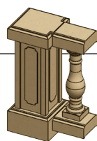
Balustrade décorative alignée avec Balustre 59 cm et trumeau TRUM59.
