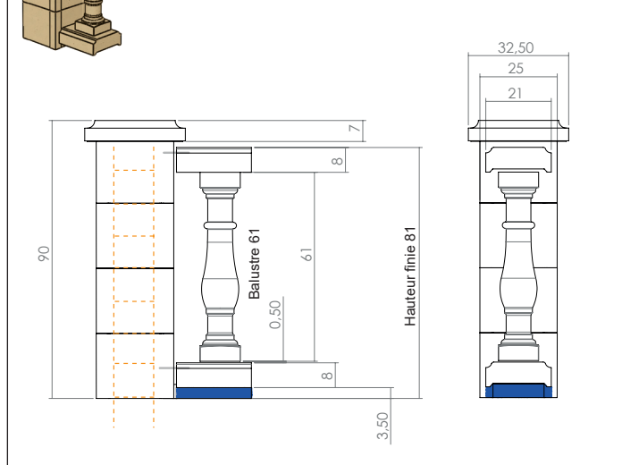
Balustrade décorative non alignée pour Balustre 59 ou 61 cm et trumeau ETRU25.
