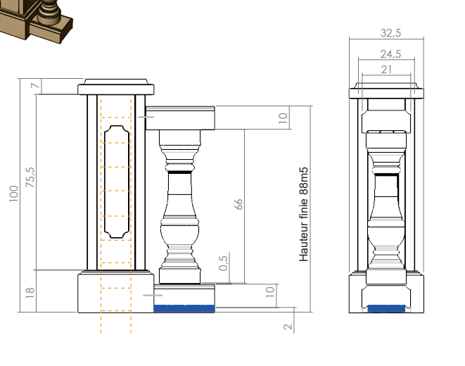
Balustrade décorative non alignée avec Balustre 66 cm et trumeau TRUM60.
