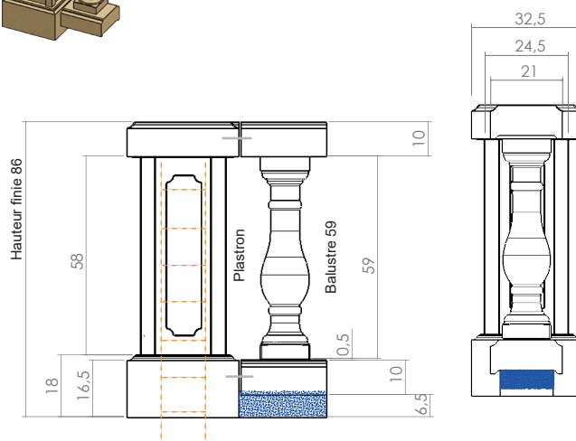
Balustrade décorative alignée avec Balustre 59 cm et trumeau TRUM59.
