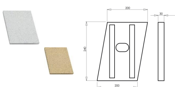
ÉLÉMENT DE LINTEAU EN PAREMENT P3 INTERMÉDIAIRE GAUCHE 200 X 240 X 30 MM
