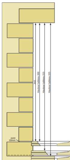
1 PAIRE DE 200 À 225 CM
