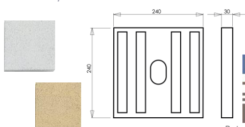
ÉLÉMENT DE JAMBAGE EN PAREMENT P6 COURT/JAMBAGE 240 X 240 X 30 MM
