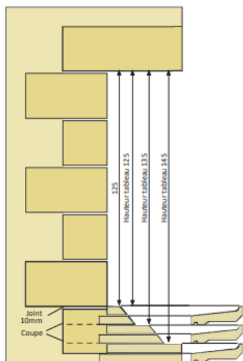
1 PAIRE DE 125 À 145 CM
