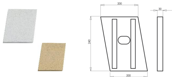
ÉLÉMENT DE LINTEAU EN PAREMENT P3 INTERMÉDIAIRE GAUCHE 200 X 240 X 30 MM
