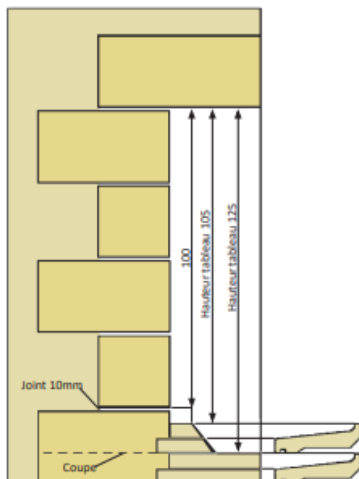
1 PAIRE DE 200 À 225 CM
