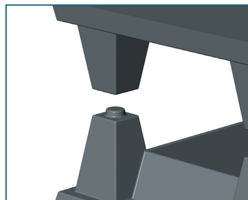
Détail de l'assemblage entre la cape et la base
