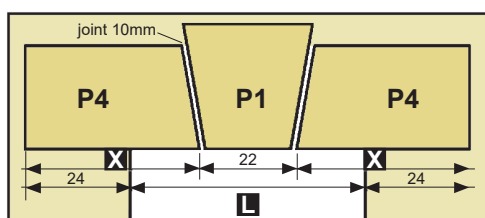
Linteau 40-60
