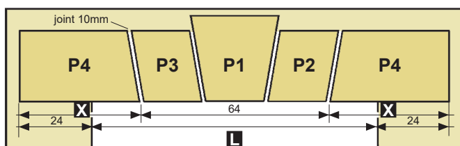
Linteau 80-100
