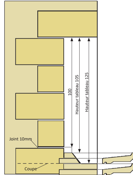
Jambage 105-125
