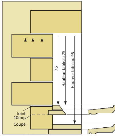
Jambage 75-95
