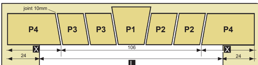
Linteau 120-140
