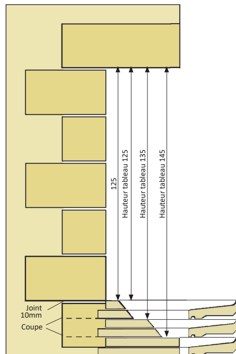
Jambage 125-145
